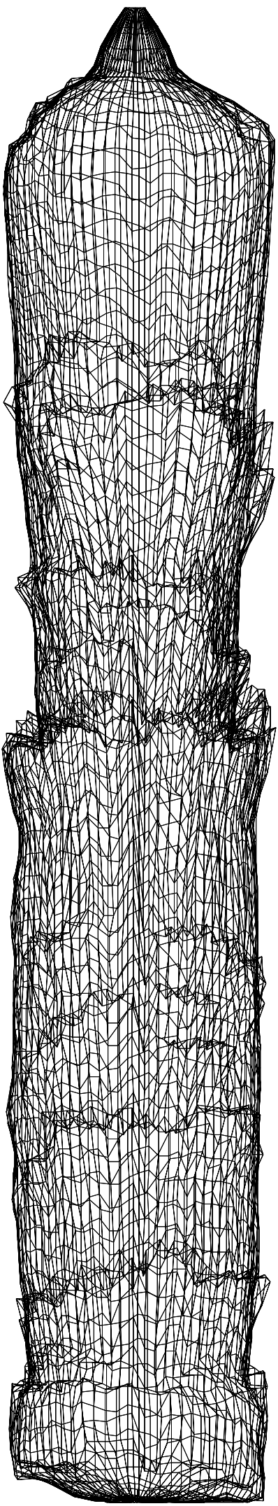
Vertikalschnitt eines 3D-Gittermodells der Kaverne Etzel K328
